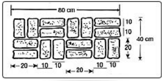
BRIQUE DESSIN «VANNERIE»
