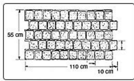
PAVÉ 10 X 10 CM
