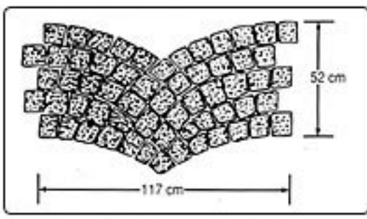
QUEUE DE PAON
